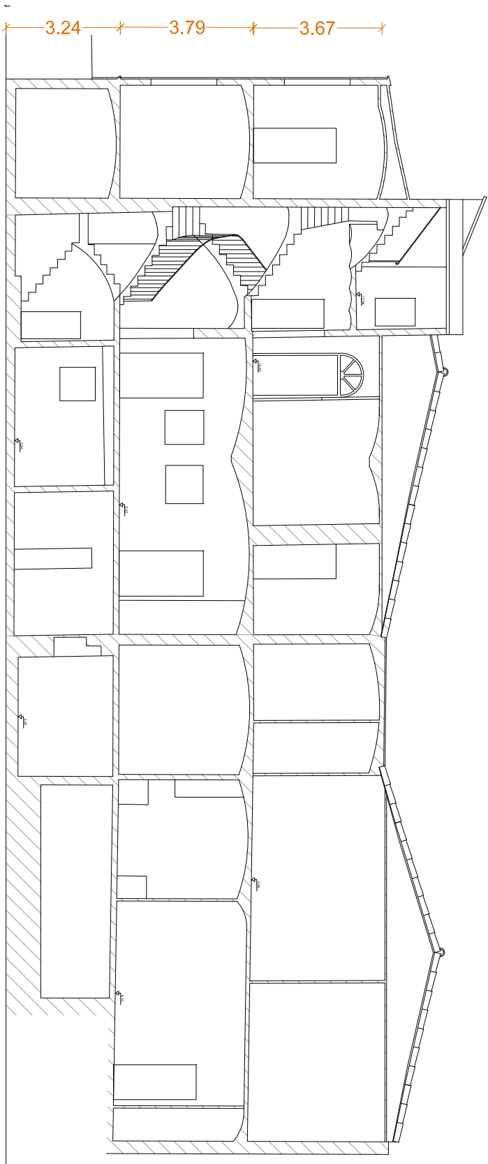
Secció BB'
